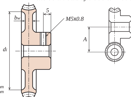
2B形 TYPE 2B
