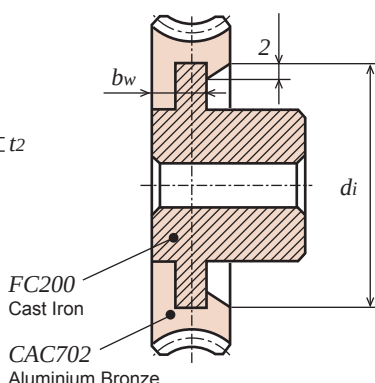
2BT1T形 TYPE 2BT1T
