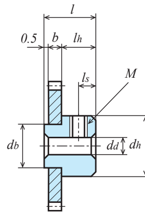
B2形 (ハブかしめ)
