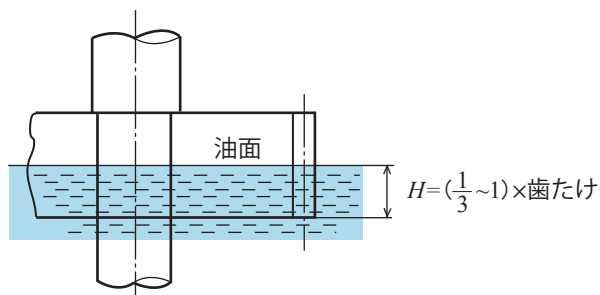
(b) 平歯車およびヘリカルギヤ（垂直軸）
