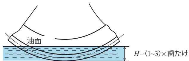
(a) 平歯車およびヘリカルギヤ（水平軸）
