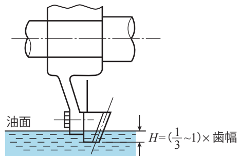
(c) かさ歯車およびハイポイドギヤ
