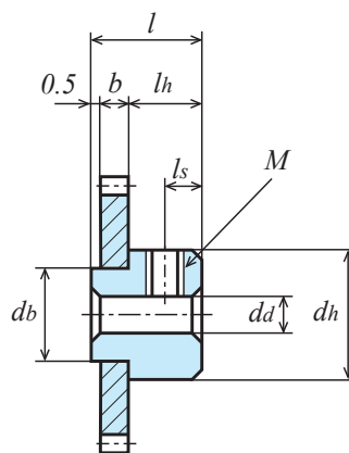
B2形 (ハブかしめ)
