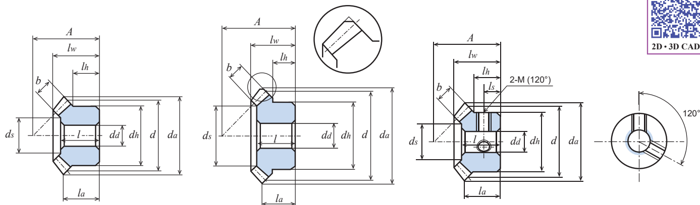
図1 (歯先面取り図)
