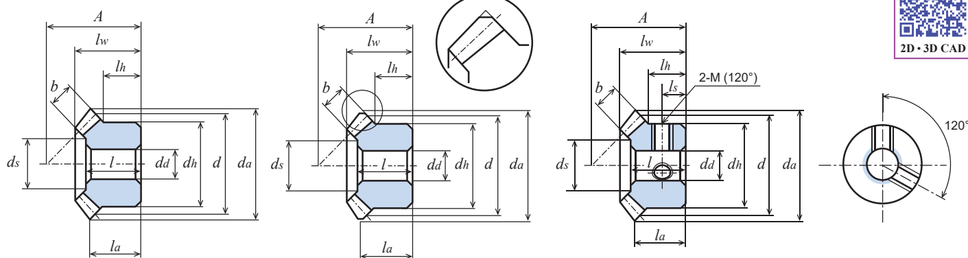
図1 (歯先面取り図)
