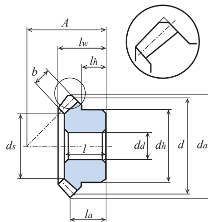
図 1 (歯先面取り図)
