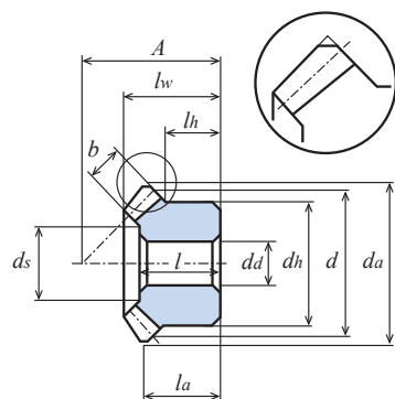
図1 (歯先面取り図)
