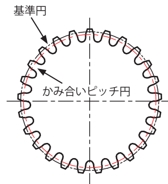
図3 負転位
