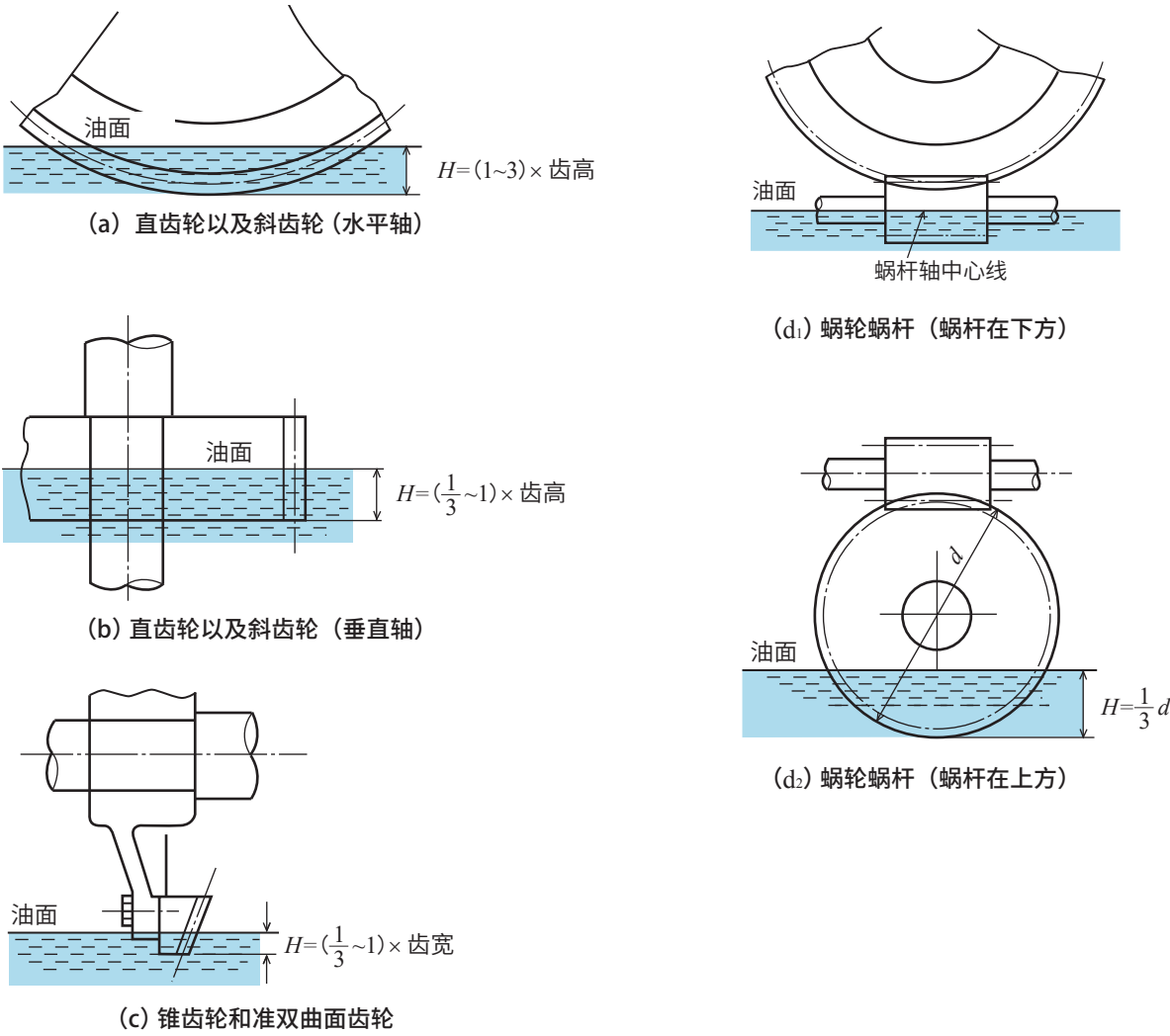
図8-1 齒車が油中に浸る量
