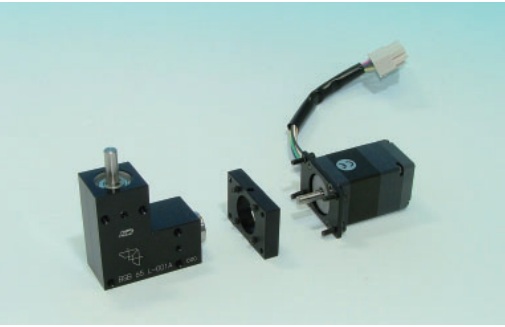
安装 B-BOX 和电机动的例子。 联结 BSB 系列齿轮箱与电机时，请使用法兰盘。
