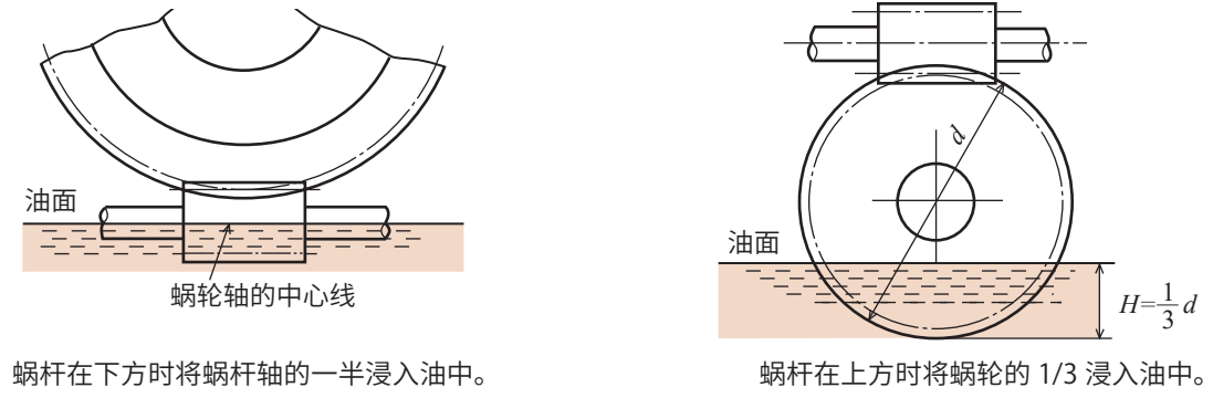
图1 润滑油量的参考值
