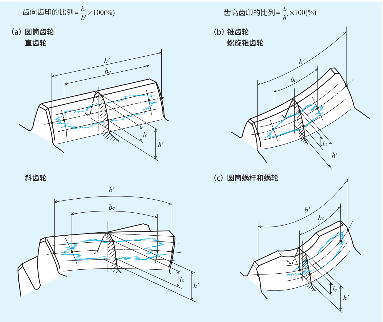
图6-1 齿轮的齿印
