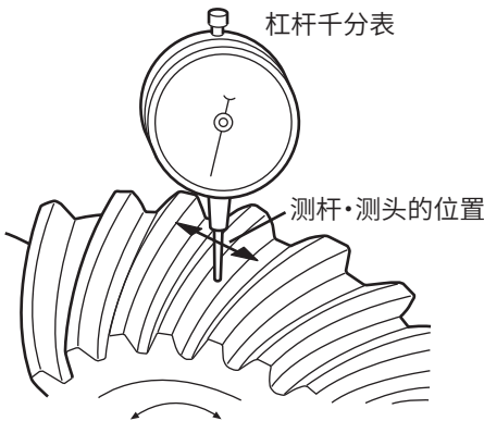
图5-1 锥齿轮侧隙的测定方法
