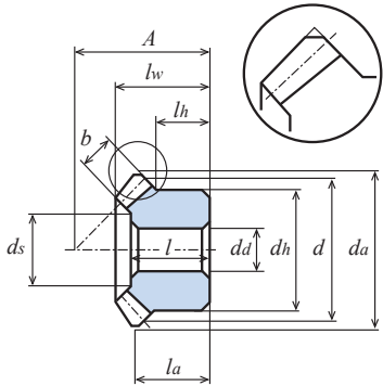
图1 (齿顶部倒角略图)
