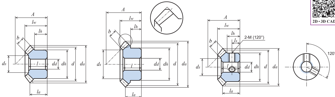
图1 (齿顶部倒角略图)
