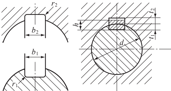
键槽横断面
