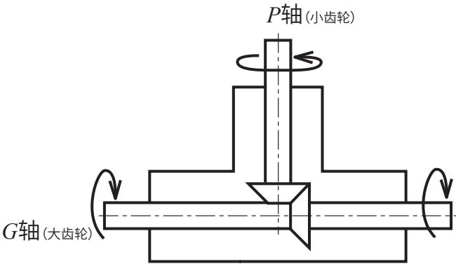
规格品 T 型
