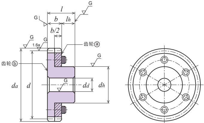
固定形状 (本图纸仅供参考)
