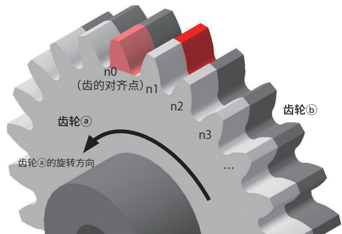
图3 节距偏移量
