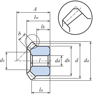
图1 (齿顶部倒角略图)
