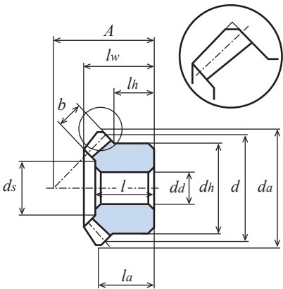
图1 (齿顶部倒角略图)
